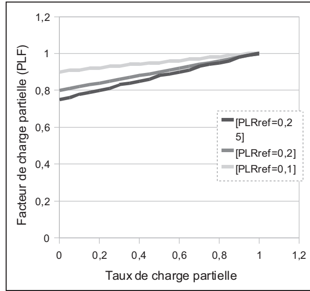
Figure 42: Modèle simplifié [PARK1977]
