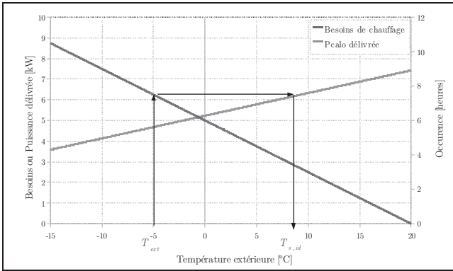
Figure 94: Température de source idéale T_{s,id} pour une température extérieure T_{ext} de 5°C
