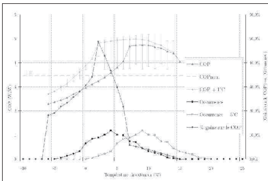
Figure 103: Gains sur le COP. Hausse de 5^\circ C de la source froide.
