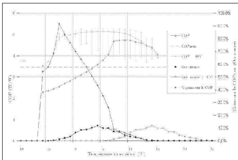
Figure 107: Hausse de 10^{\circ}C de la température de la source. Impact sur le COP.
