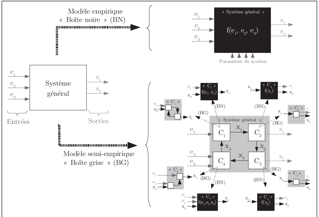
Figure 29: Possibilités de modélisation par « approche inverse »
