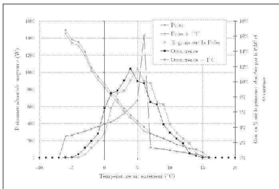
Figure 98: Gains sur la puissance absorbée par la PAC dus à l'élévation de 1^\circ C de la source froide
