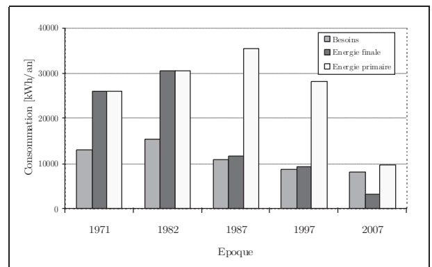
Figure 129: Consommation en énergie primaire pour les différents états de la maison
