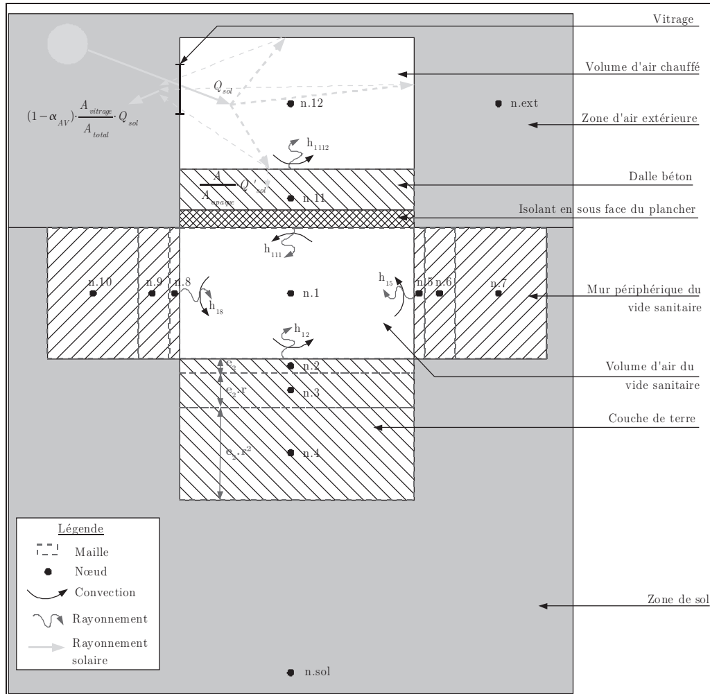
Figure 72: Maillage et bilan thermique du vide sanitaire
