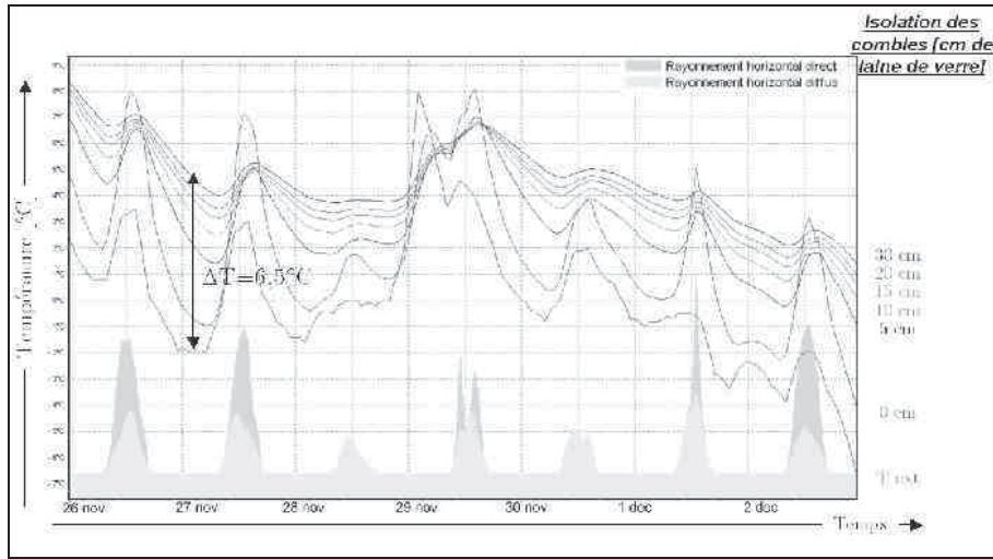
Figure 76: Évolution des températures intérieures du comble perdu d'un volume de 19 m 3 , en fonction de l'isolation de la sous-pente de toit au climat de Trappes
