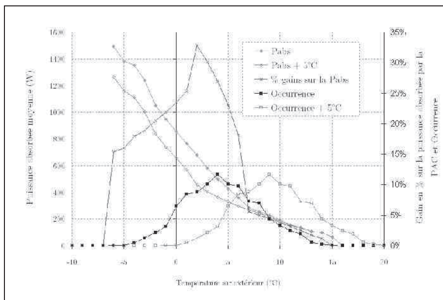
Figure 102: Gains sur les consommations de la PAC. Hausse de 5^\circ C de la source froide.
