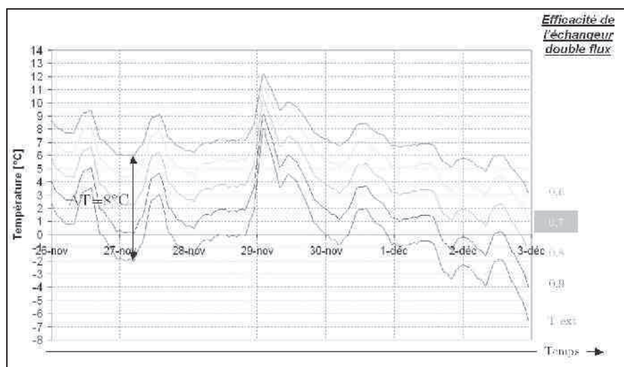
Figure 80: Évolution de température de l'air extrait à la sortie d'une ventilation double flux, pour différente valeur d'efficacité de l'échangeur, au climat de Trappes
