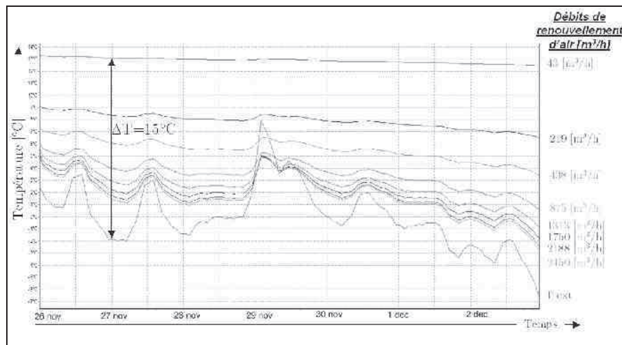
Figure 73: Évolution de la température d'un vide sanitaire au climat de Trappes pour différents taux de renouvellement d'air
