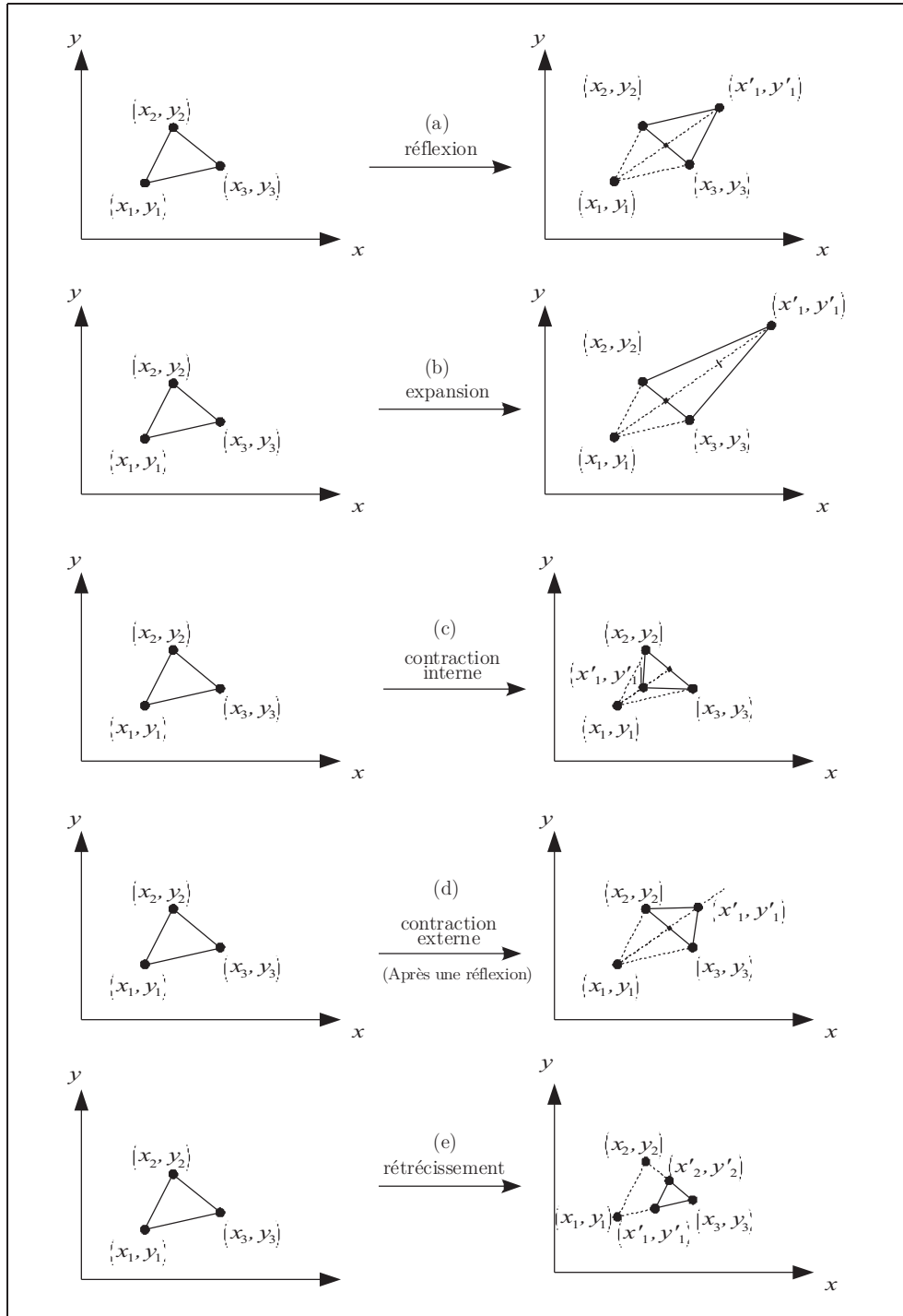
Figure 56: Transformation du simplexe proposé par la méthode d'optimisation de Nelder-Mead
