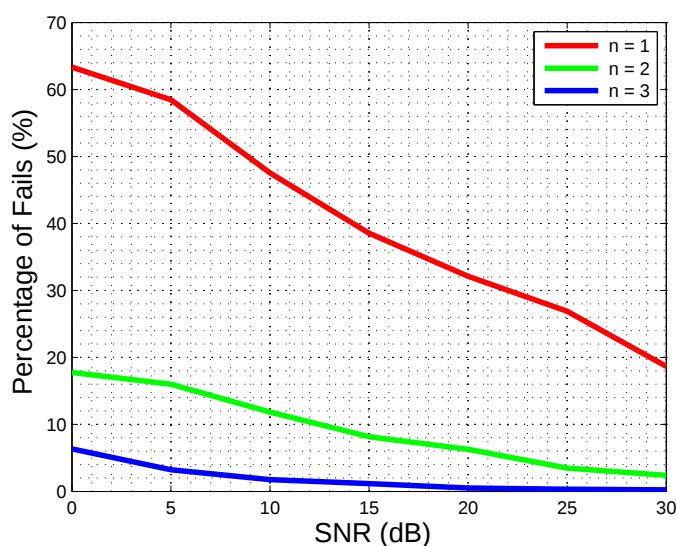
Figure C.8: Résultat de performance de domaine temporel PD(D)P-F en fonction de n .
