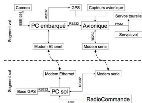
FIG. 1.34 – Le drone Lhasa lors de son vol de recette en Mai 2005, et architecture matérielle embarquée.
