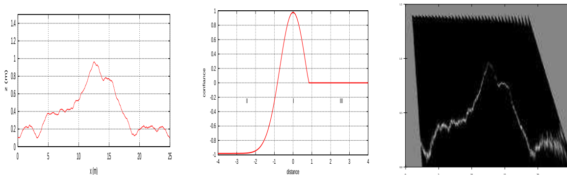
FIG. 1.16 – Illustration en 2 dimensions d’une méthode de mise à jour d’une grille d’occupation à partir de données de profondeur, en utilisant les formules de mise à jour des probabilités de Dempster-Shafer. Un profil de terrain simulé (à gauche) est perçu par une caméra stéréoscopique ”plane”, dont le modèle d’erreur est illustré au centre. La figure de droite montre la grille d’occupation construite en intégrant les données d’une quarantaine de positions de la caméra (qui s’est déplacée horizontalement au dessus du profil). Grâce à la fusion d’un très grand nombre de points, les erreurs résultantes sont inférieures à 2.0 cm, alors que dans cette simulation l’écart type sur l’estimation de la distance est de 0.1x^2 , x étant la distance des points perçus.
