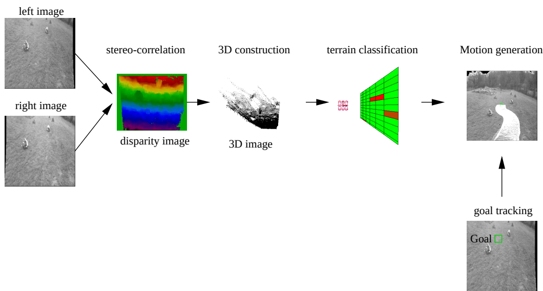
FIG. 1.21 – Principe de la génération de mouvements par la méthode des potentiels.
