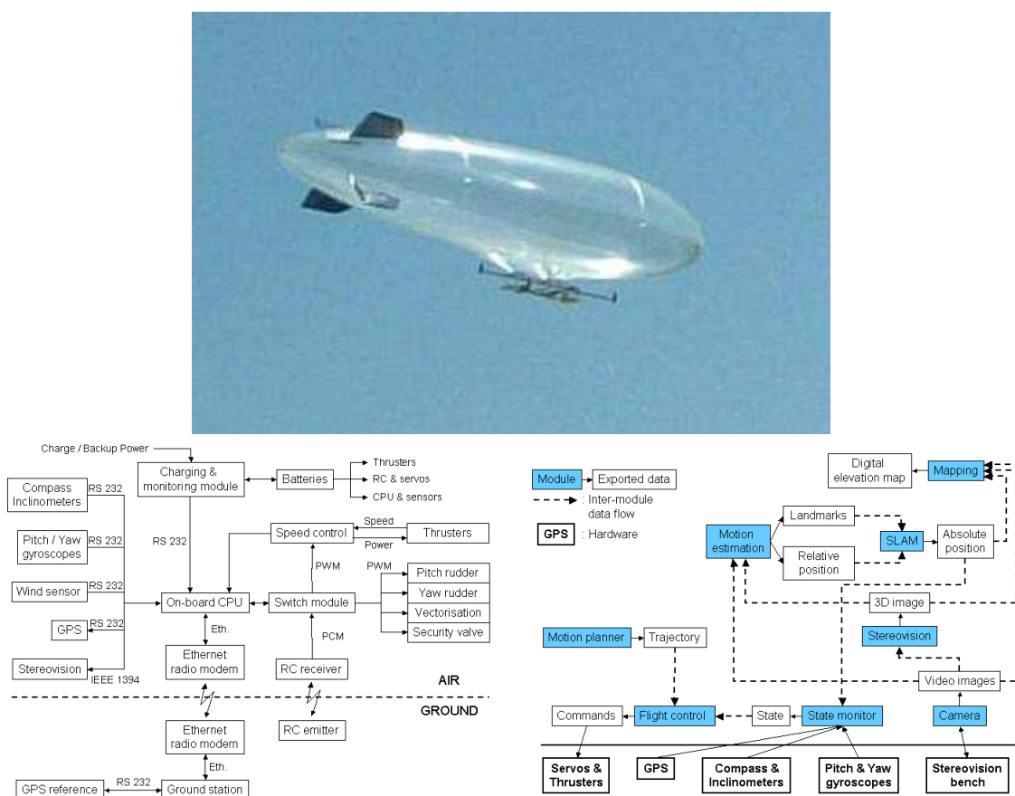
FIG. 1.33 – Dernière version du ballon dirigeable Karma. En bas : architectures matérielle et logicielle embarquées.
