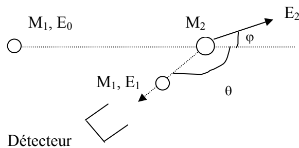
Figure 2.10 : Principe de la RBS
