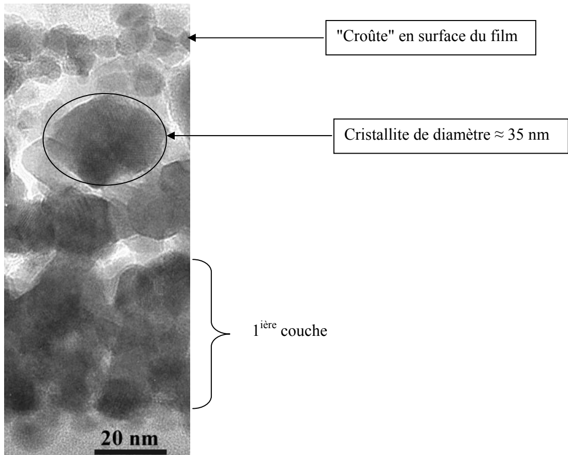
Figure AIV. 9: Image MET à plus fort grandissement du film 4 couches recuit CTA à 600°C.
