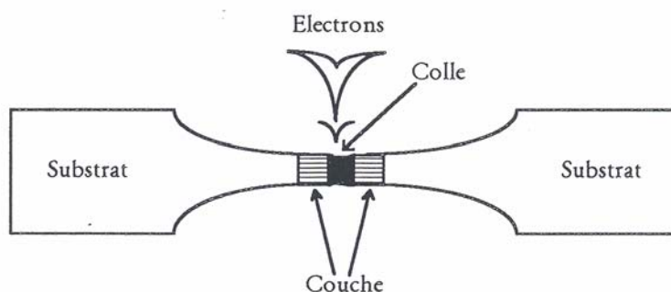
Figure AII.9 : Etapes de l'assemblage des échantillons pour une coupe- transverse.
