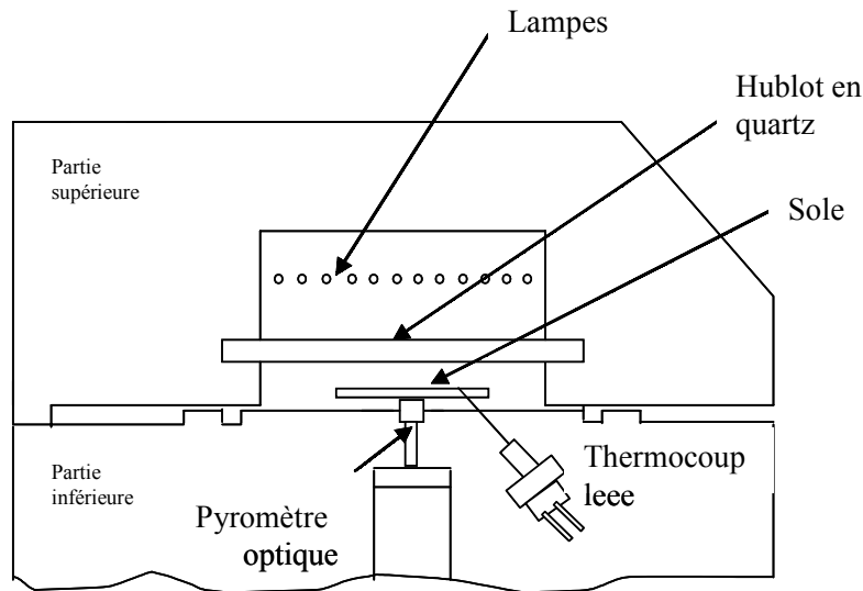
Figure AII.3 : Vue générale du four RTA
