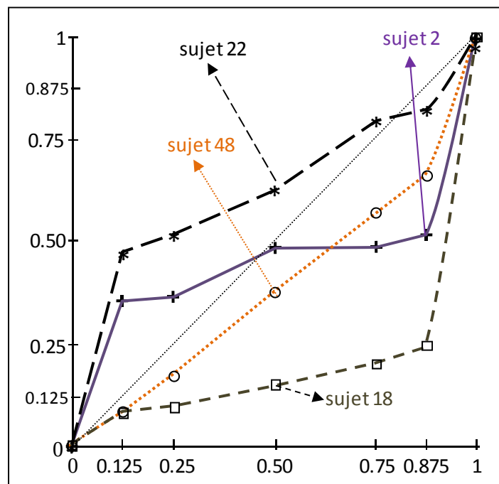
Graph 0.4.5 : Transformations de probabilité pour la température à Paris
