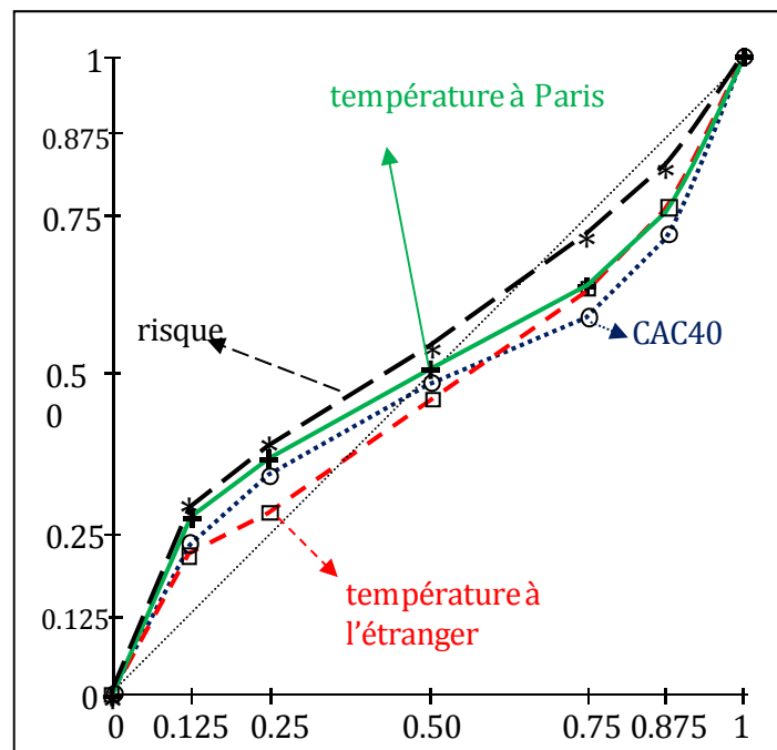
Graph 0.4.4 : Transformations de probabilité moyennes pour le groupe Réel
