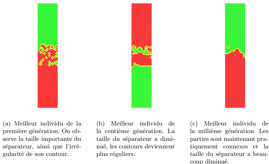
FIG. 4.1: Exemple de résultats obtenus sur une grille 2D avec un partitionnement utilisant un algorithme génétique seul, sans multi-niveaux ni heuristiques d'optimisation locale. Le résultat obtenu n'est pas celui de l'algorithme utilisé dans PT-SCOTCH ; il s'agit juste d'une mise en évidence d'une convergence, même avec des critères lâches.
