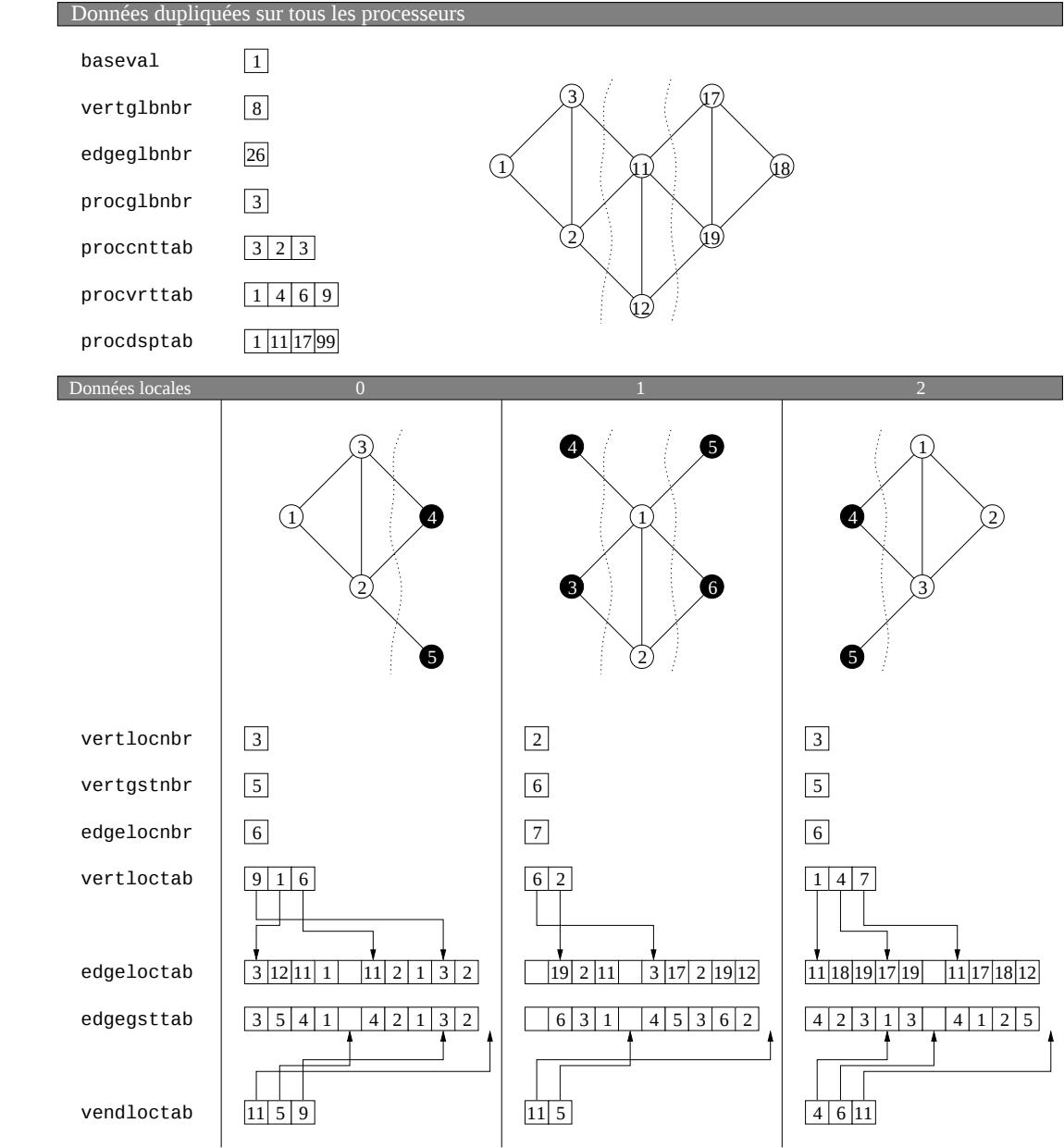
FIG. 1.16: Exemple de distribution des données sur 3 processeurs dans le cas d'un graphe avec une numérotation à trous.
