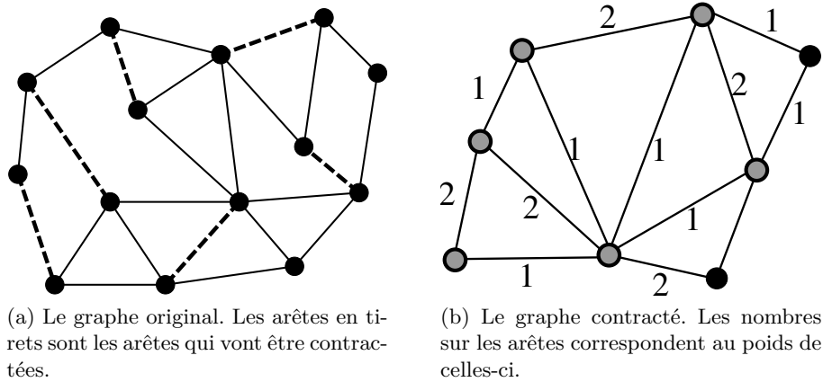
FIG. 1.9: Exemple de contraction de graphe par appariement d'arêtes.
