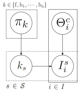
FIGURE 2 – Modèle graphique : I_i^s , La couleur de la projection dans la vue i de l'échantillon s , dépend des modèles couleurs \Theta_i^c et de l'étiquette k_s . \pi_k représente les coefficients de mélange.
