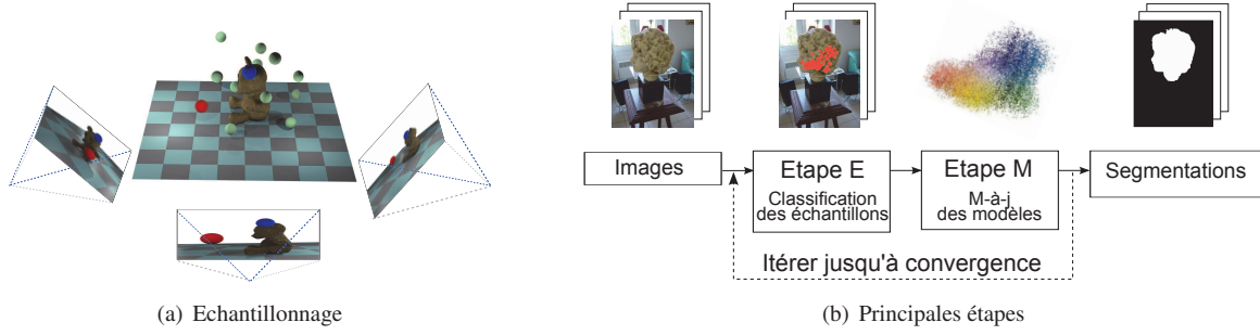
FIGURE 1 – Aperçu global de la méthode : (a) Les échantillons sont représentés par des sphères en 3D pour une bonne visualisation. L'échantillon bleu est étiqueté "objet" car il se projette dans la région avant-plan dans toutes les vues. L'échantillon rouge est étiqueté "fond", car deux caméras le classent dans l'arrière-plan. (b) Schéma algorithmique : la méthode itère entre classification des échantillons et mise à jour des modèles. Une segmentation finale est effectuée pour transférer la classification éparse des échantillons vers une classification dense des pixels.
