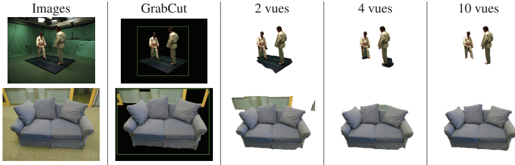
FIGURE 7 – Comparaison avec une approche monoculaire (GrabCut) et influence du nombre de vues sur le résultat de segmentation sur les séquences Art martiaux et Couch .
