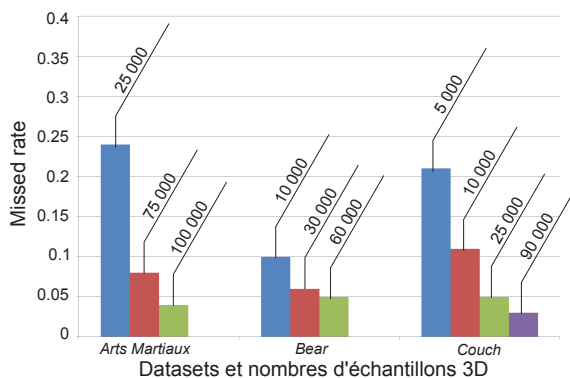
FIGURE 11 – Résultats avec différents nombre d'échantillons 3D. Le taux de pixels étiqueté "fond" à tort ( Missed rate ) est utilisé comme mesure d'erreur.
