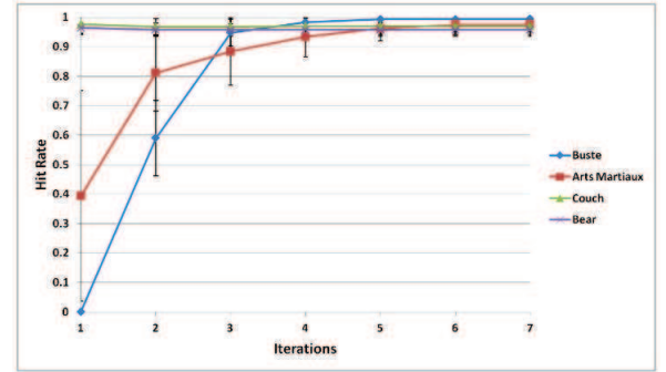
FIGURE 9 – Pour les 4 jeux de données, l'algorithme converge après 6 itérations.
