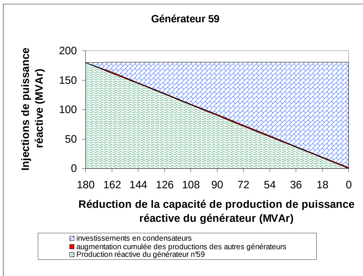
Figure 24 : injections de puissance réactive en remplacement de la production du générateur n°59 pour un niveau de charge du réseau de 10000 MW
