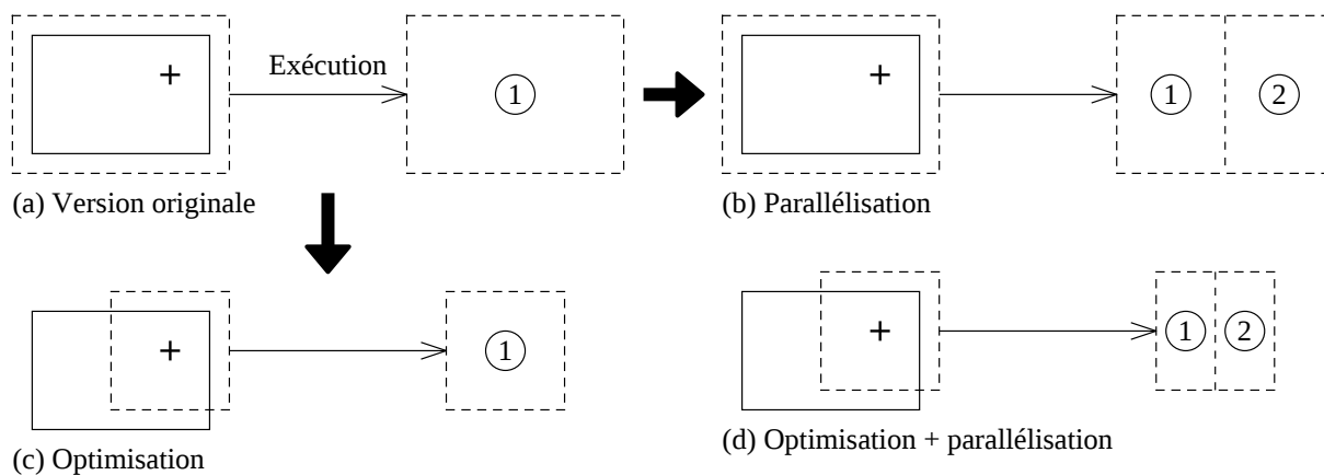
FIGURE 2.1 – (a) L'implémentation originale utilise la totalité ( rectangle en pointillés ) des interactions de l'espace ( rectangle en trait continu ) en un point donné ( croix ). (b) La parallélisation permet l'exécution parallèle de la fonction (intégration/interpolation) sur deux sous-ensembles par deux processeurs (① et ②). (c) L'optimisation au niveau du code source permet de ne sélectionner que les interactions les plus adaptées. (d) Avec l'optimisation et la parallélisation cumulées, on remarque que l'exécution parallèle s'opère sur des sous-ensembles restreints, le temps d'exécution en est donc doublement réduit.
