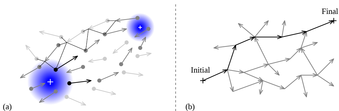
FIGURE 3.1 – Alors que les connexions sont explicites dans un graphe (b), elles résultent de propagations ( pointillés ) dans l'espace d'interaction (a). Alors que la coordination implicite de cette thèse met à jour un champ d'activité afin de décider de la prochaine décision à prendre en continu, les algorithmes de recherche ordonnée déterminent dans le graphe un chemin unique et discret. Alors que le graphe est plus ou moins statique, le champ d'activité est modifié en permanence. En particulier, les notions de début et de fin, ici grossièrement équivalentes aux interactions ( croix blanche et diffusion bleue ) sont dynamiques.
