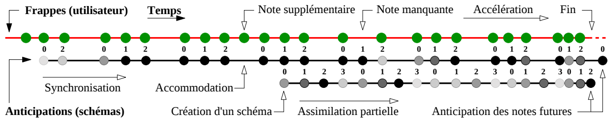
FIGURE 5.6 – Capture annotée du programme de TamTam dans sa deuxième version. Les chiffres indiqués au dessus de la ligne des anticipations correspondent au numéro de la cellule la plus active dans le rythme associé. Ici sont combinés le nouvel algorithme de synchronisation et l'apprentissage de rythmes nouveaux par variation/sélection. Cette visualisation à l'avantage de faire apparaître les futures notes anticipées au fur et à mesure de l'interaction avec l'utilisateur.
