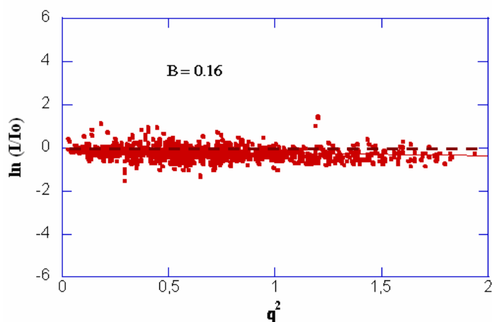
Figure 2.25 : Graphique de Wilson (comparaison des données à 150 K et à 138 K).
