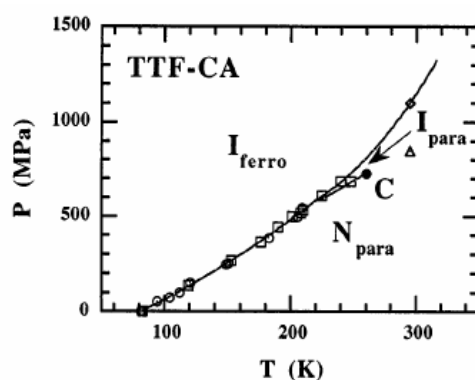
Figure 4.2 : Diagramme de phase du complexe moléculaire à transfert de charge TTF-CA. (Lemée-Cailleau (1997)).
