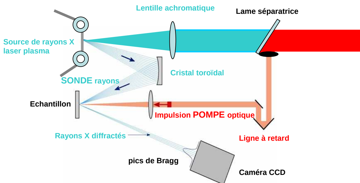
Figure 4.18 : Schéma du dispositif pompe optique sonde X mis en place au LOA.
