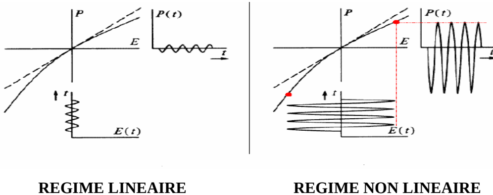
Figure 3.10 : Partie linéaire et non linéaire de la polarisation en fonction du champ électrique.
