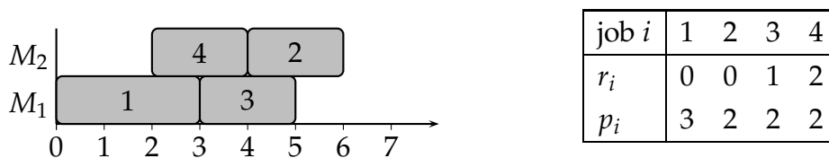
Figure 2.1 – Exemple d'ordonnancement semi-actif.
