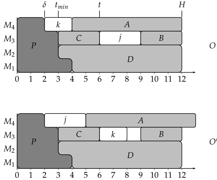
Figure 2.17 – Ordonnancements O et O' lorsque j et k sont sur deux machines différentes.
