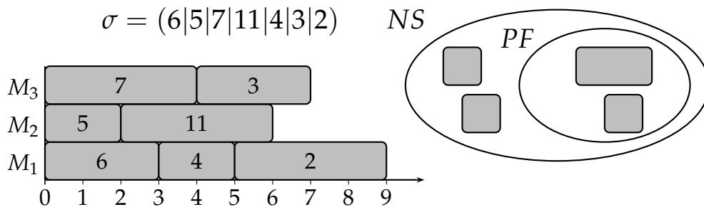
Figure 4.2 – Représentation d'un sommet de l'arbre de recherche.
