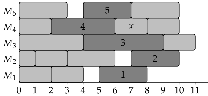
Figure 2.3 – Les jobs \{1, 2, 3, 4, 5\} forment le front d'adjacence du job x .
