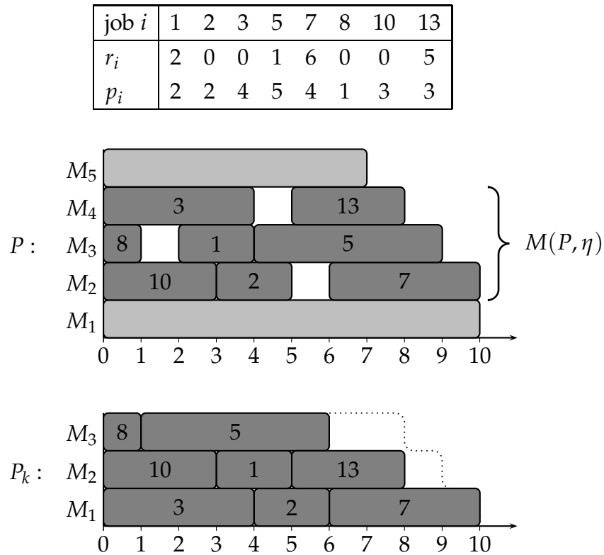
Figure 2.9 – Exemple de dominance selon la règle RD_k .
