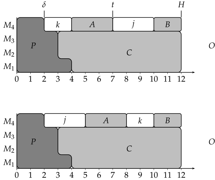
Figure 2.12 – Ordonnancements O et O' lorsque j et k sont sur la même machine.
